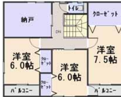
2階平面図
