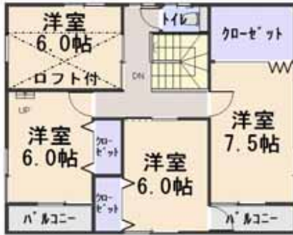
2階平面図
