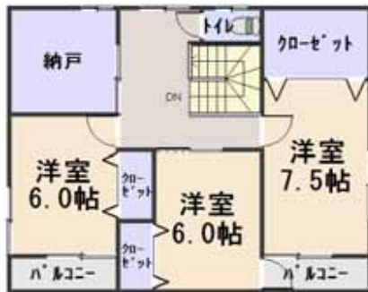
2階平面図
